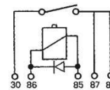
MINI RELE CON DIODO 12V 40A
